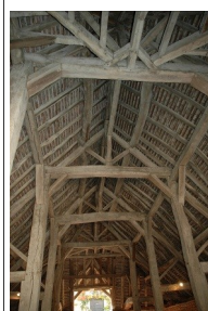
La charpente des halles de Brancion
